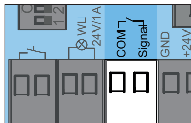
Abb. 7: Anschlussklemme für eine 2-Draht-Lichtschanke
