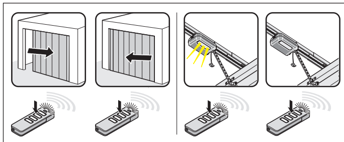
Abb. Impulsfolge für
