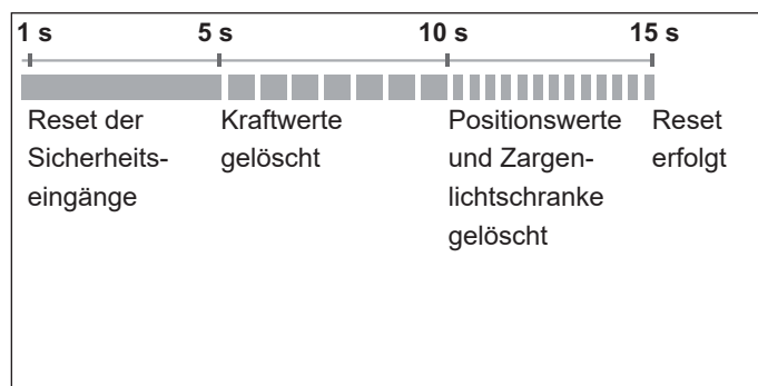
Abb. Übersicht der Zeitabfolge der Status-LED am Laufwagen beim Drücken des grünen Reset-Tasters
