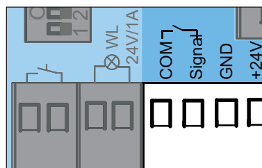
Abb. 8: Anschlussklemme für eine 4-Draht-Lichtschanke
