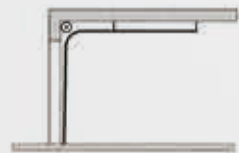
Normalbeschlag Sturzbedarf 220mm, Seitenanschlag 90mm (Alu 100mm) Normal installation Lintel requirement 220mm, side inset 90mm (Alu 100mm)
