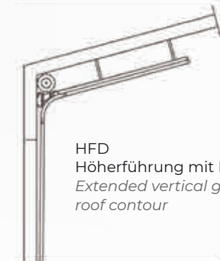
NID Niedrigsturzbeschlag mit Dachfolge Low lintel fitting parallel to roof contour
