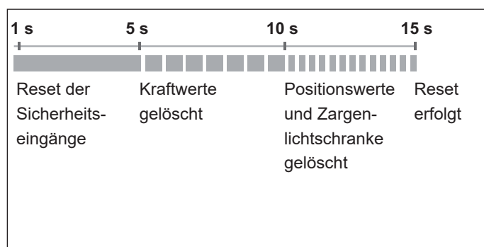
Abb. Übersicht der Zeitabfolge der Status-LED am Laufwagen beim Drücken der grünen Reset Taste
