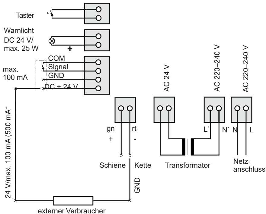
Abb. Anschlussplan Wandsteuerung
