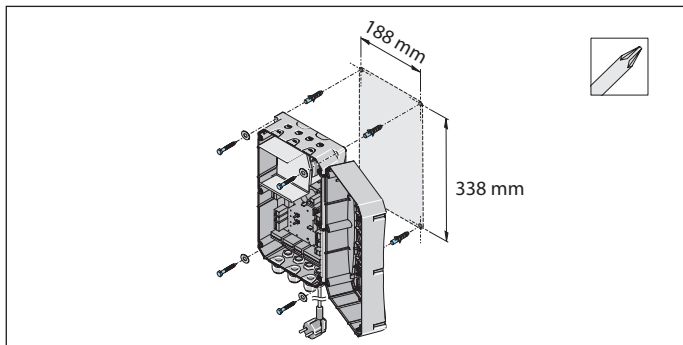
Abb. 3: Montagebeispiel
