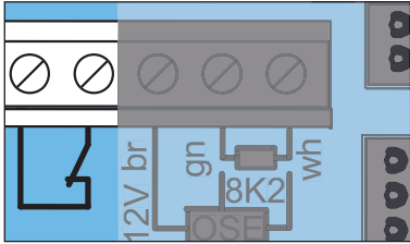
Abb. Anschluss Schlupftürsicherung
