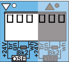
Abb. Anschluss Sicherheitskontaktleiste OSE für Tor ZU
