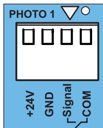
Abb. Anschluss 4-Draht-Lichtschanke, LED orange
