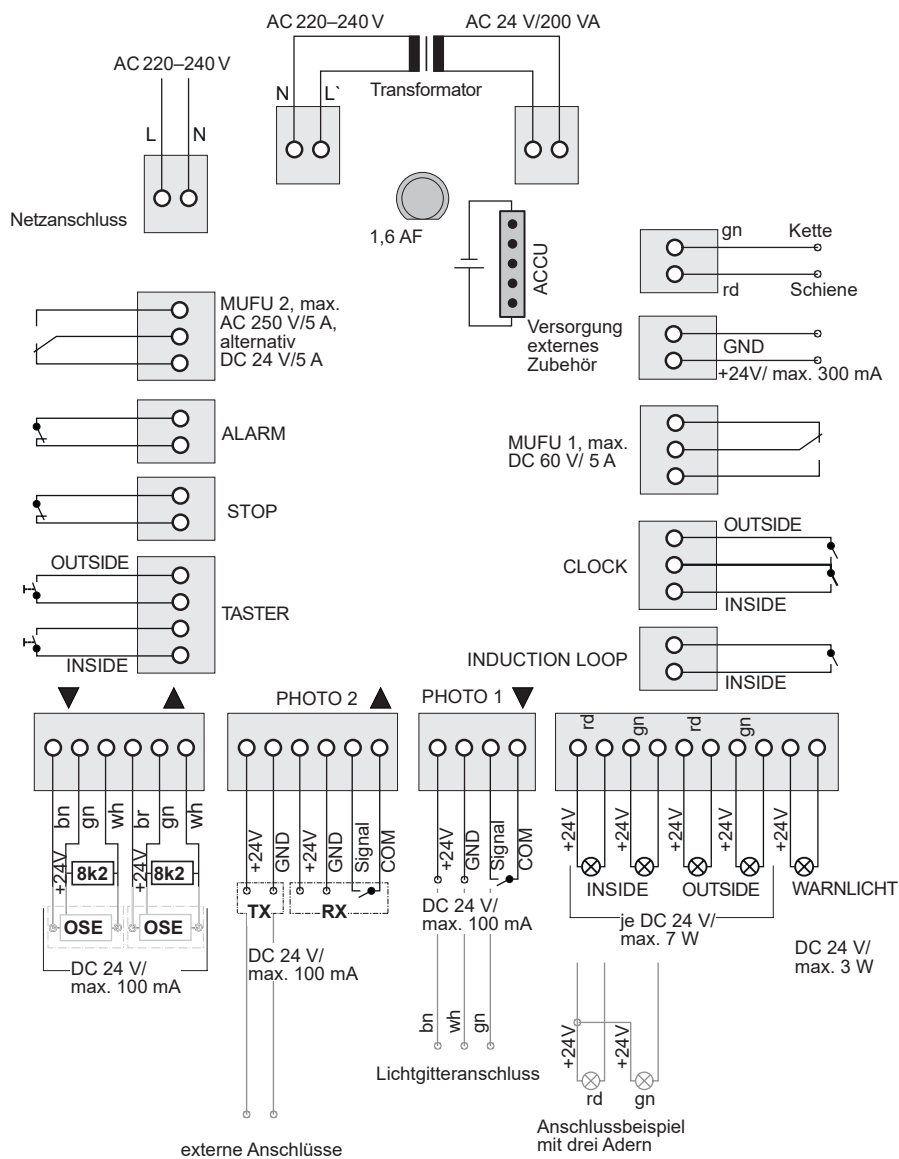
Abb. Anschlussplan Wandsteuerung
