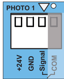
Abb. Anschluss Lichtgitter für Tor ZU
